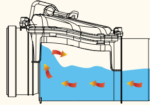
Activation du Système Anti-Retour Contre les Eaux Pluviales & Usées
